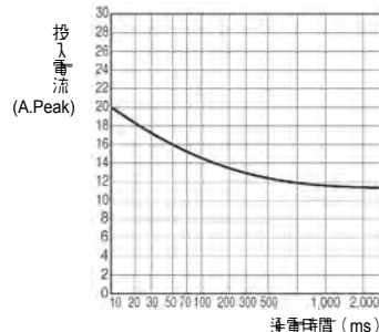
G3NA-D210B 型
