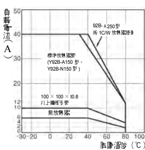
G3NA-440B 型
