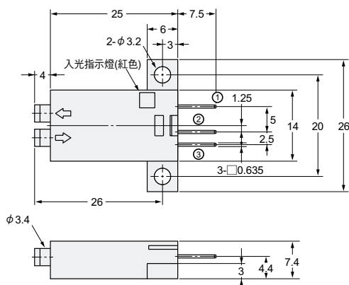
端子配置
