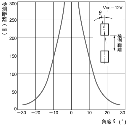
EE-SPW321/421型
