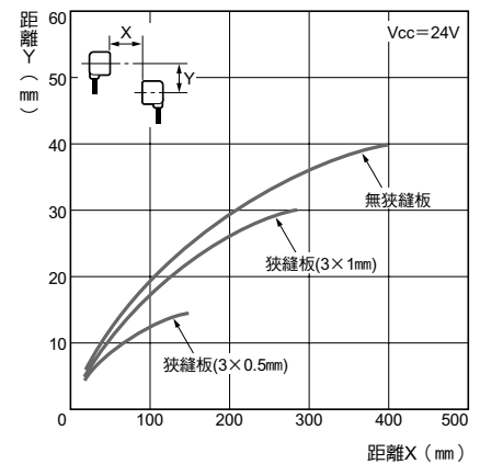
移動平均特性 EE-SPW321/421型
