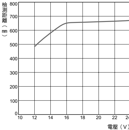
EE-SPW321/421型
